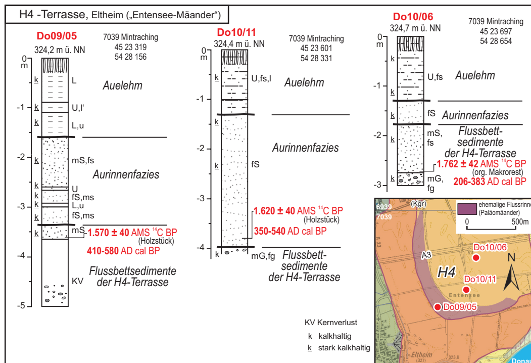
Abb. 8: 14 C-Alter organischer Makroreste aus den obersten Flusssanden des H4-Mäanderbogens in der Flur „Entensee“ mit Profilschnitt ( 14 C-Alter in Tab. 2, Kartengrundlage: Top. Karte 1:25 000 © Bayerische Vermessungsverwaltung 2009).
