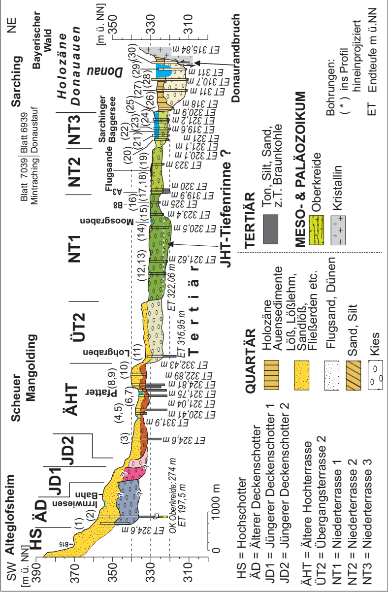
Beilage 2: Geologischer Profilschnitt Min1 von Alteglofsheim über Mangolding und Mintraching nach Sarching. Zur Lage des Profils siehe Beilage 1. Die Herkunft der Bohrungen ist in Beilage 5 zusammengestellt.
