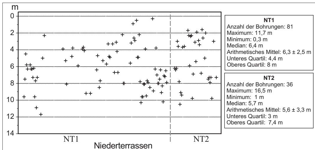
Abb. 7: Mächtigkeit des Kieskörpers (m) im Bereich der Niederterrassen NT1 und NT2 der Donau auf Blatt 7039 Mintraching zusammengestellt nach Schichtverzeichnissen von Bohrungen.
