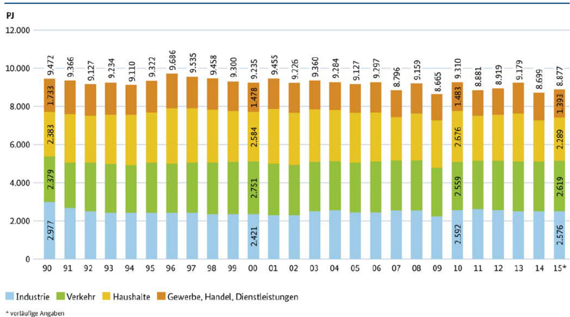
Abbildung 7: Entwicklung des Endenergieverbrauchs nach Sektoren
